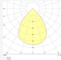
Curva fotométrica 90° Photometric Curve 90° Curva fotométrica 90°
