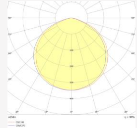
Curva fotométrica 120° Photometric Curve 120° Curva fotométrica 120°
