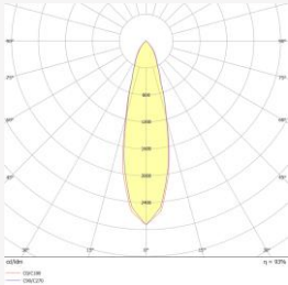
Curva fotométrica 30° Photometric Curve 30° Curva fotométrica 30°
