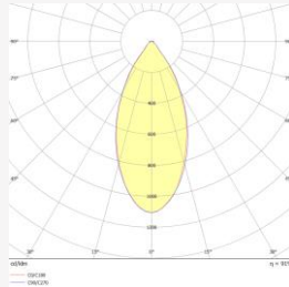
Curva fotométrica 60° Photometric Curve 60° Curva fotométrica 60°
