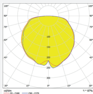
Curva fotométrica 120°
