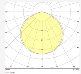
Curva fotométrica 120°
