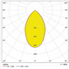
Curva fotométrica 30°
